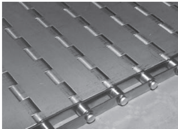
Voorbeeld van SC-RK dichte scharnierplattenband met rollenkant
