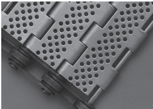
Voorbeeld van een SC-HK scharnierplattenband met zijketting en perforatie
